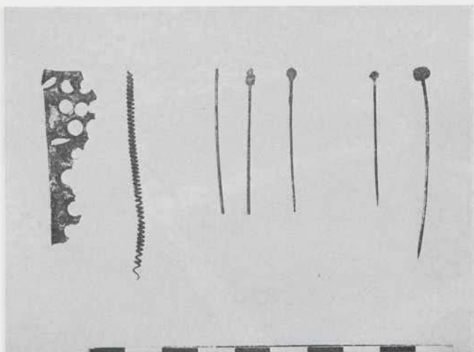
Afb. 24 Dordrecht. De productiegang in een 14-eeuwse speldenmakerij. Overblijfselen gevonden in een van de 'werkplaatsen'. Links een plaatje koperblik waaruit de schijfjes voor de koppen gestansd worden en in een spiraal opgedraaid koperdraad. Midden het maken van de kop aan een eindje recht afgesneden koperdraad. Rechts spelden met aangevijlde scherpe punt. Foto ROB.
