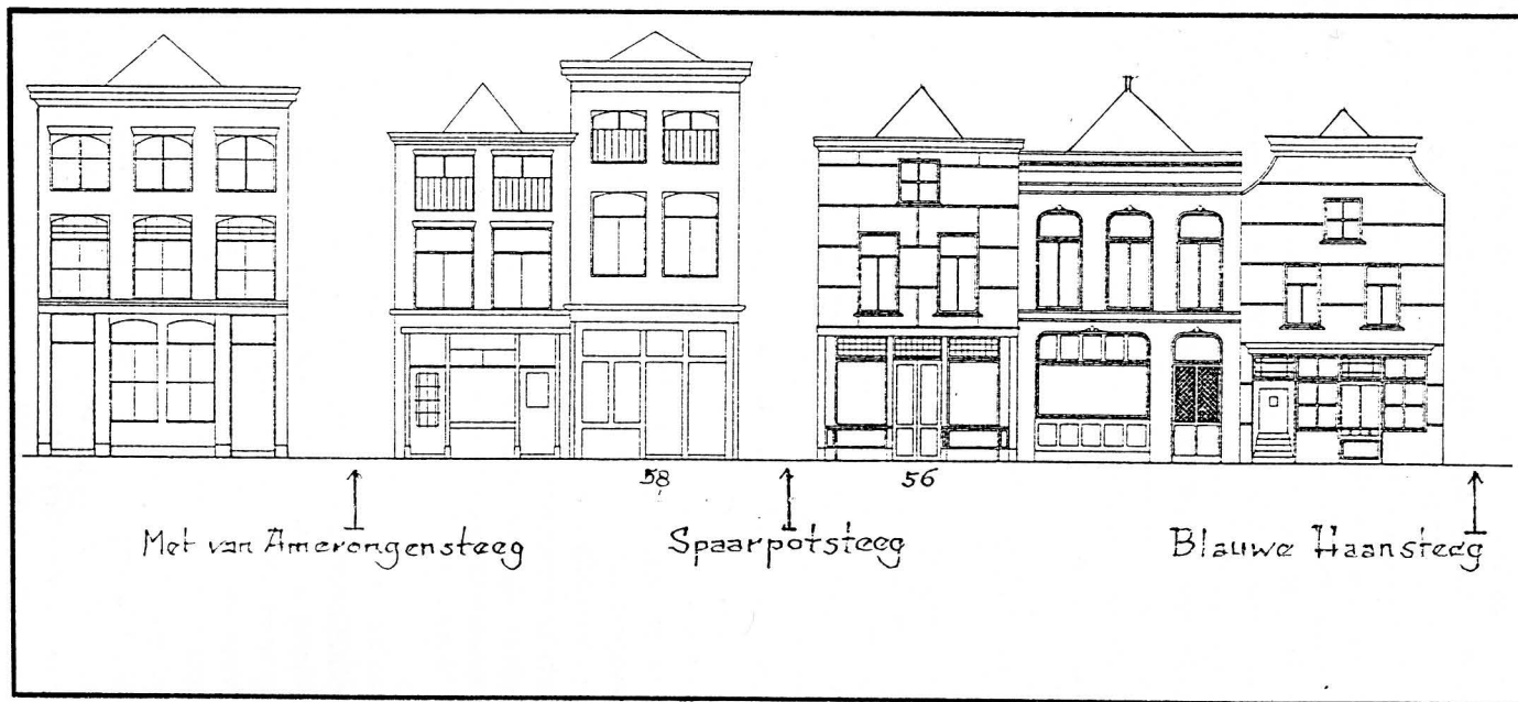
De huizenwand Kalkhaven nr. 52 t/m 64. De huizen in opstand getekend naar de toestand in 1948.
