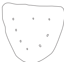
hak met houtpennen gevormd door vier lagen leer
