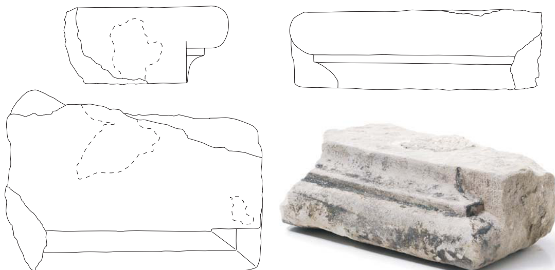
Afb. 32: Zijaanzichten en bovenaanzicht van het sierlijstfragment (V44). Schaal 1:4. De foto toont het object ondersteboven ten opzichte van de positie waarin het oorspronkelijk ingemetseld is geweest.
