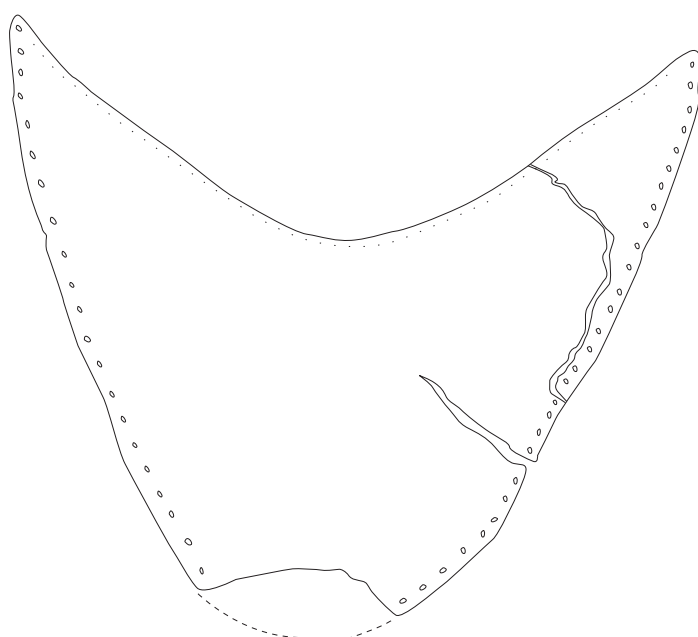
hak met houtpennen gevormd door vier lagen leer
