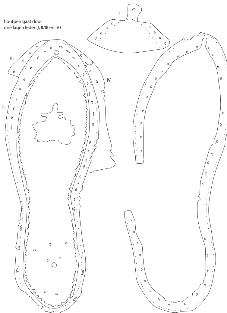
Afb. 69: Complete schoenzolen. Links: V45-L01, onder: V45-L05. Schaal 1:2. Tekenaar: T. Busch.
