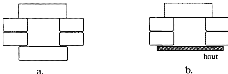
Schematische doorsnede van de watergoten ten noorden van het huis van Paffenrode, afm. baksteen 24 x 12 x 5 cm
